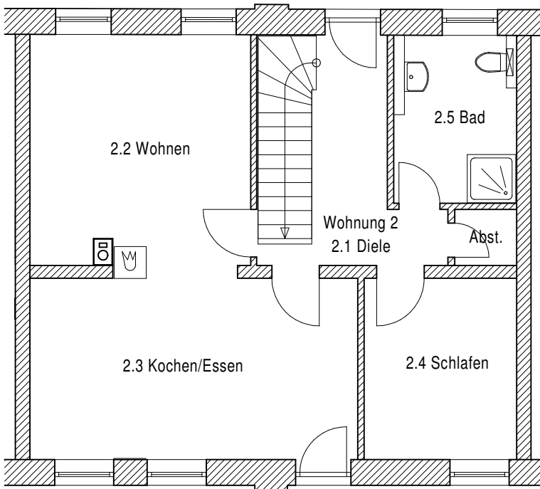
Erdgeschoss
