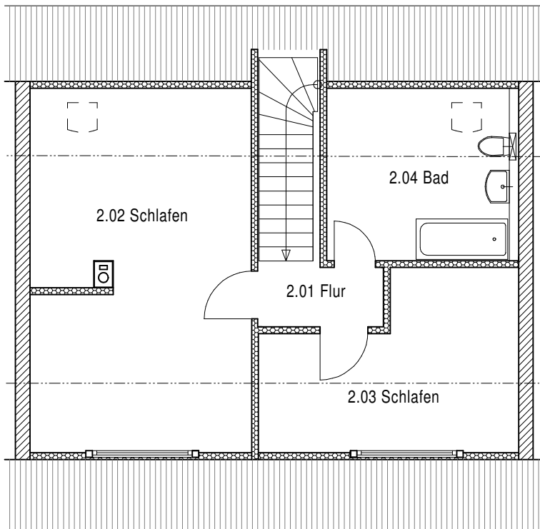
Dachgeschoss
